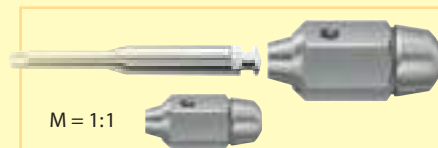
Отвёртка короткая
