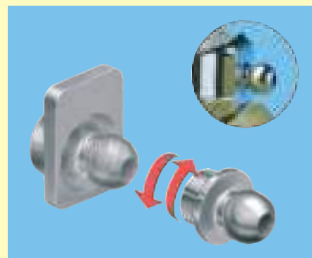
vks-sg 1,7 / 2,2 взаимозаменяемые сферы
