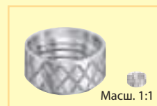
Резбовая втулка Титан 2,2 2 шт. № 450 0007 6
