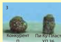
При 300°C пластмасса-конкурент показывает отчетливое расширение. Пи-Ку-Пласт ХП 36, напротив, уменьшается в объёме.
