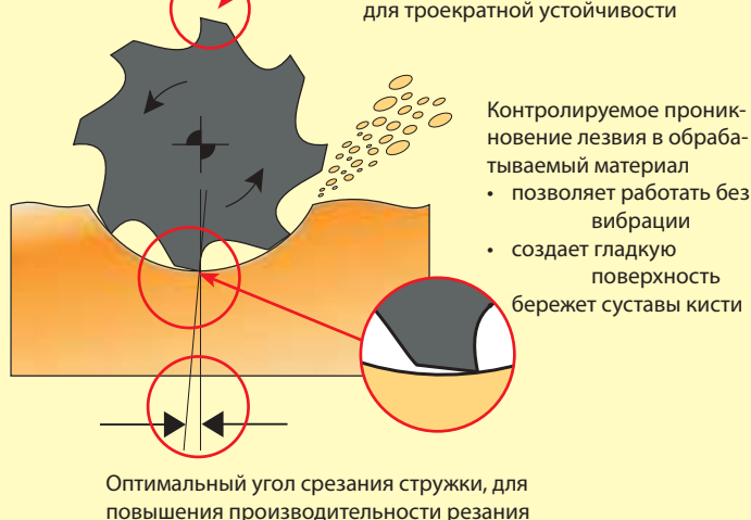
Инструмент Бредент с Интершлифом
